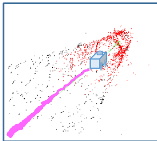
カメラ画像による位置推定 position estimation using camera images
