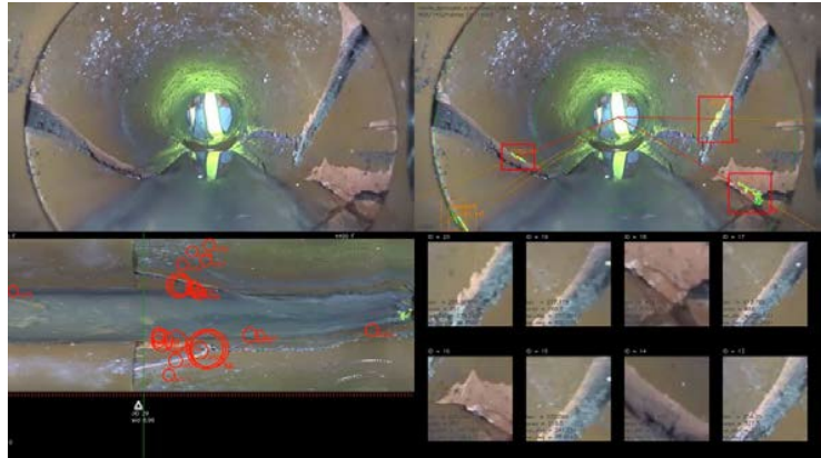
パイプ検査ソフト（異常検出） pipe inspection software (anomaly detection)
