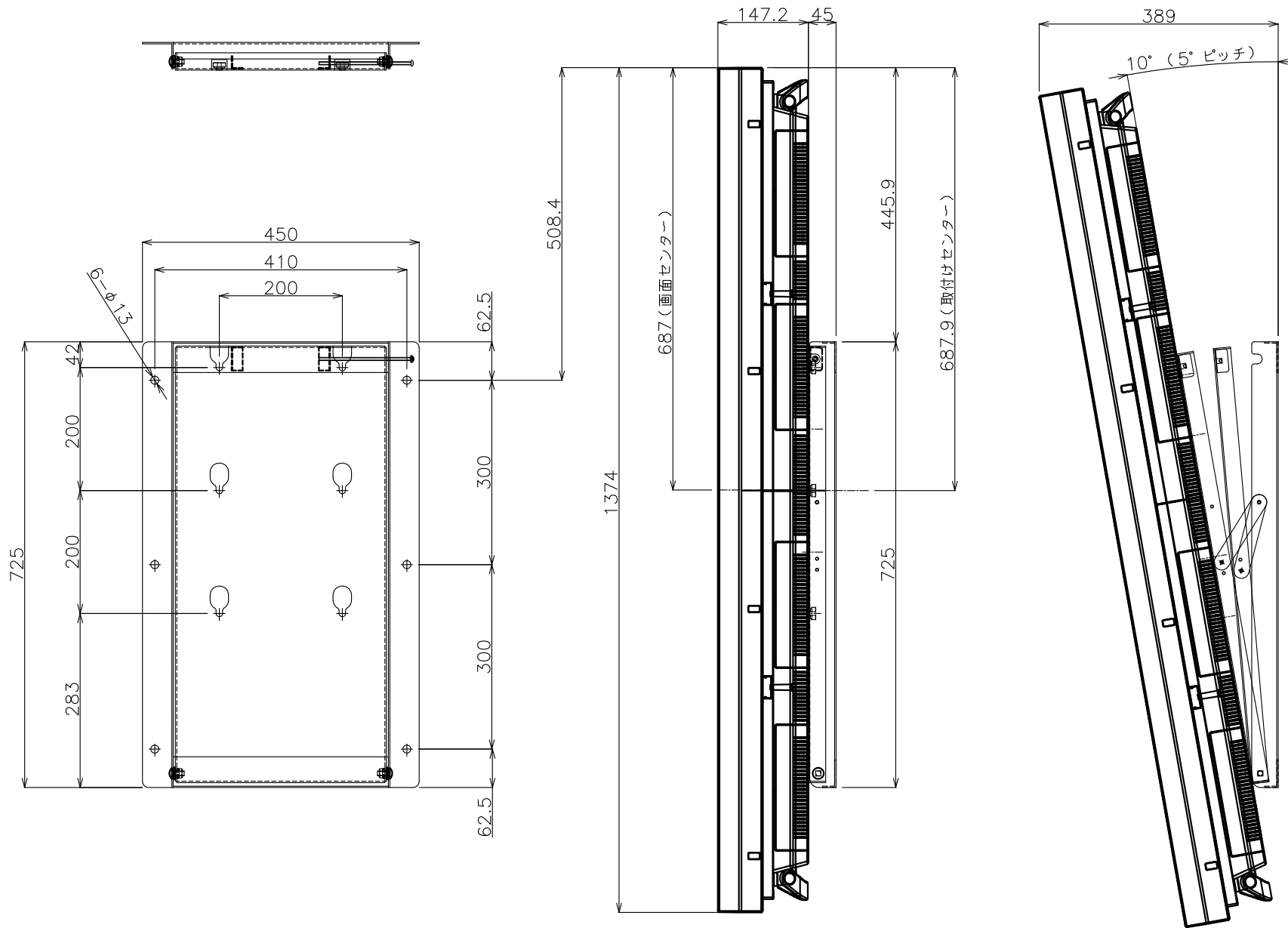
壁掛け金具 (PN-A601取付時) PN-ZK602 外観図
