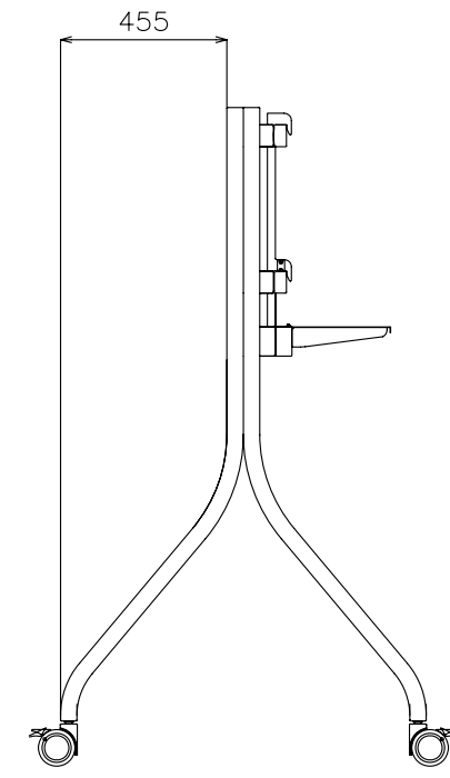
フロアスタンド PN-ZS70F 外観図
