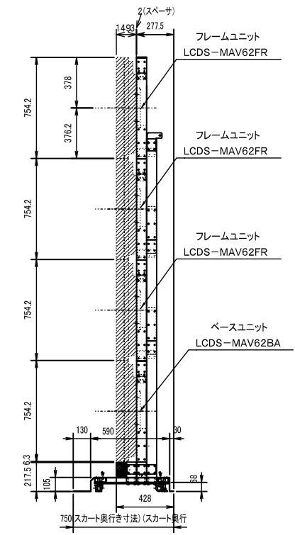
マルチディスプレイフロアスタンド (横取付4段4列) LCDS-MAV62BA, LCDS-MAV62FR LCDS-MAV60JO 3ユニット組立時 外観図
