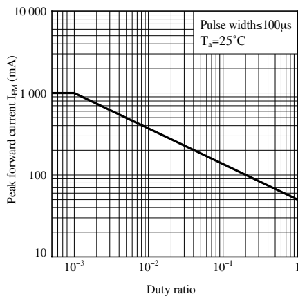
Fig.5 せん頭順電流 デューティ比
