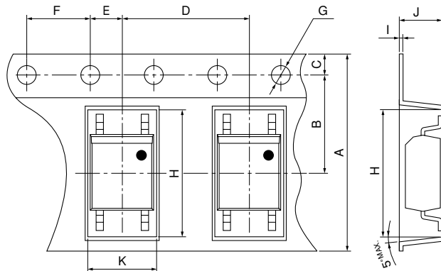
寸法表
