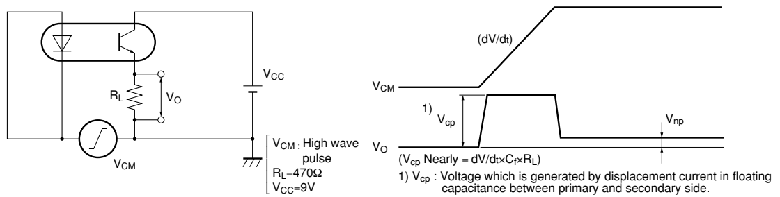
Fig.1 同相除去電圧の測定回路
