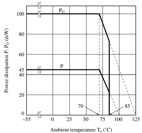
Fig.4 許容損失低減曲線
