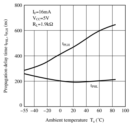
Fig.10 伝搬遅延時間—周囲温度特性
