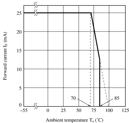
Fig.3 順電流低減曲線
