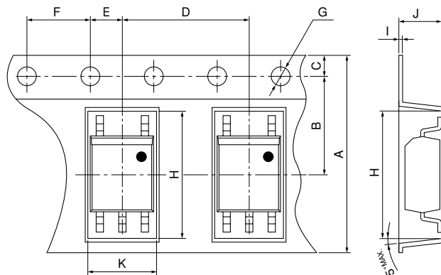
寸法表
