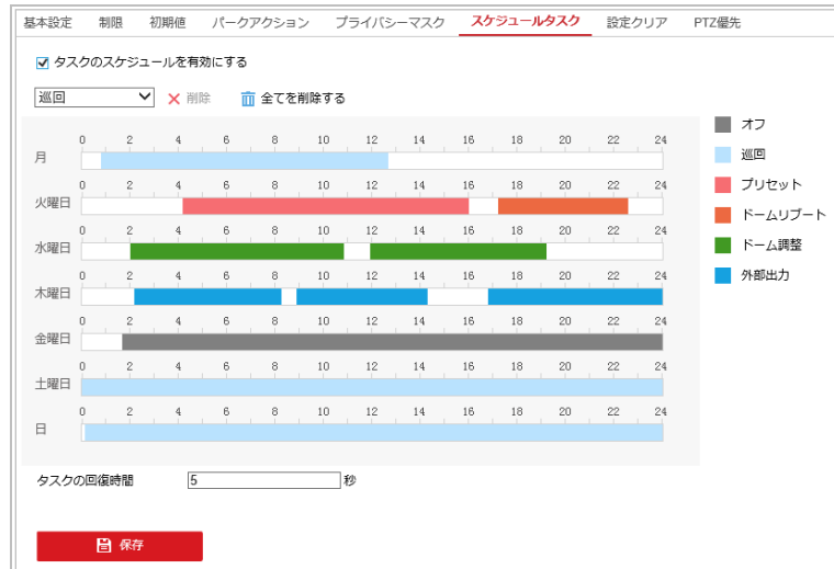
図 9-11 スケジュールとタスク種別の編集
