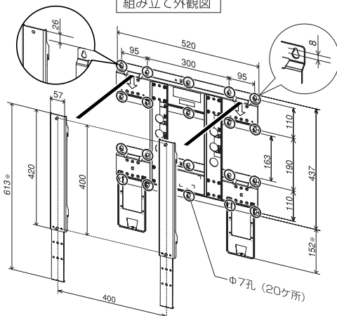
組み立て外観図
