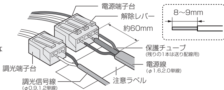
電源線・調光信号の接続例(保護チューブを使用する場合)
